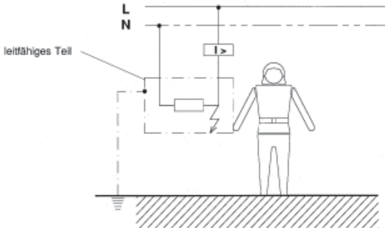
Bild 5 Fehlerstromschutz
